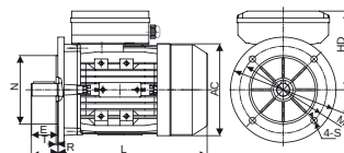
Figure 2 IM B5
