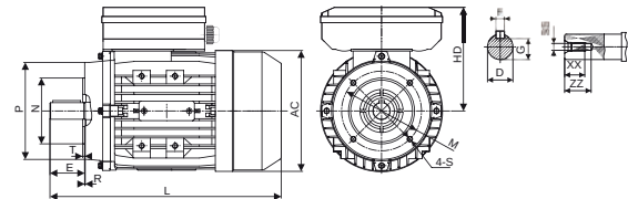
Figure 3 IM B14
