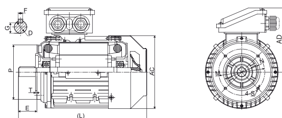
Figure 4 IM B14
