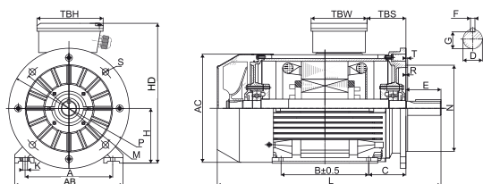
Figure 2 IM B35
